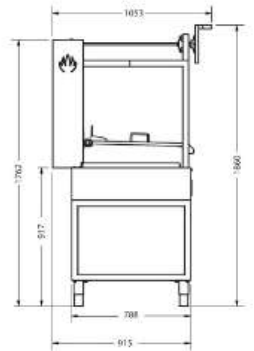
VUE LATÉRALE
