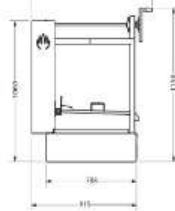
VUE LATÉRALE
